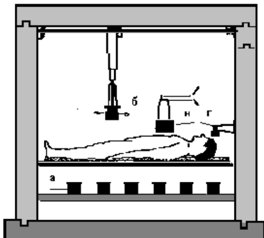
Рис. 5.1. СИЧ экспертного класса, геометрия измерения “лежа”
