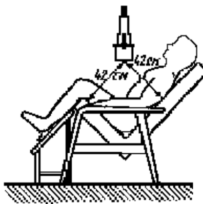
Рис. 5.2. Геометрия измерения “стандартное кресло”
